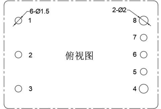
推荐PCB开槽尺寸
